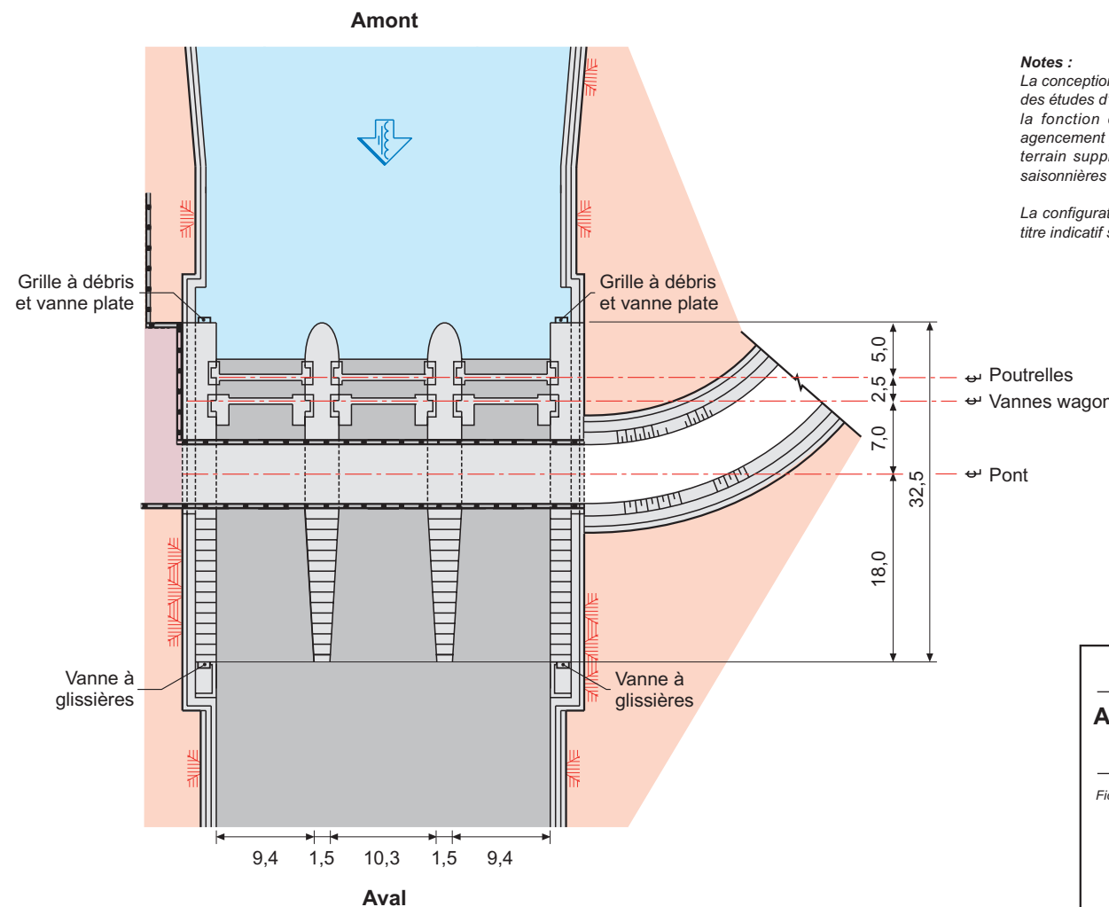
Évacuateur de crues – Vue en plan
