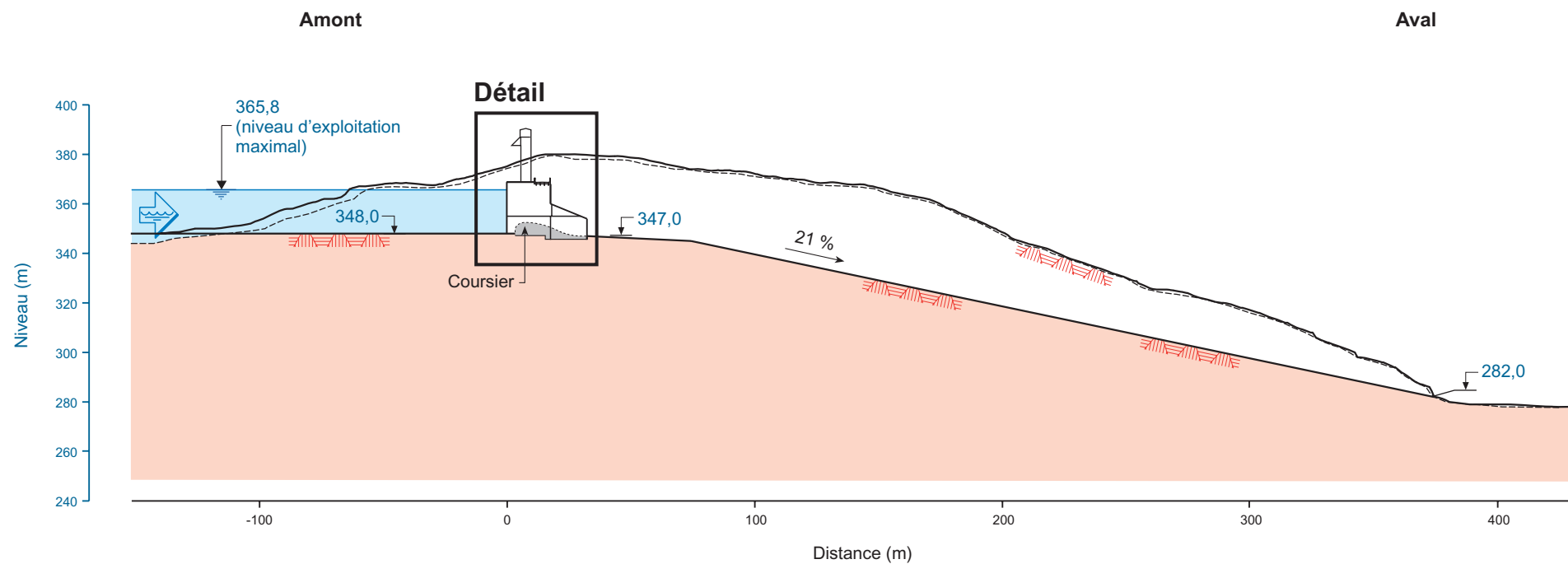
Évacuateur de crues – Profil longitudinal A
