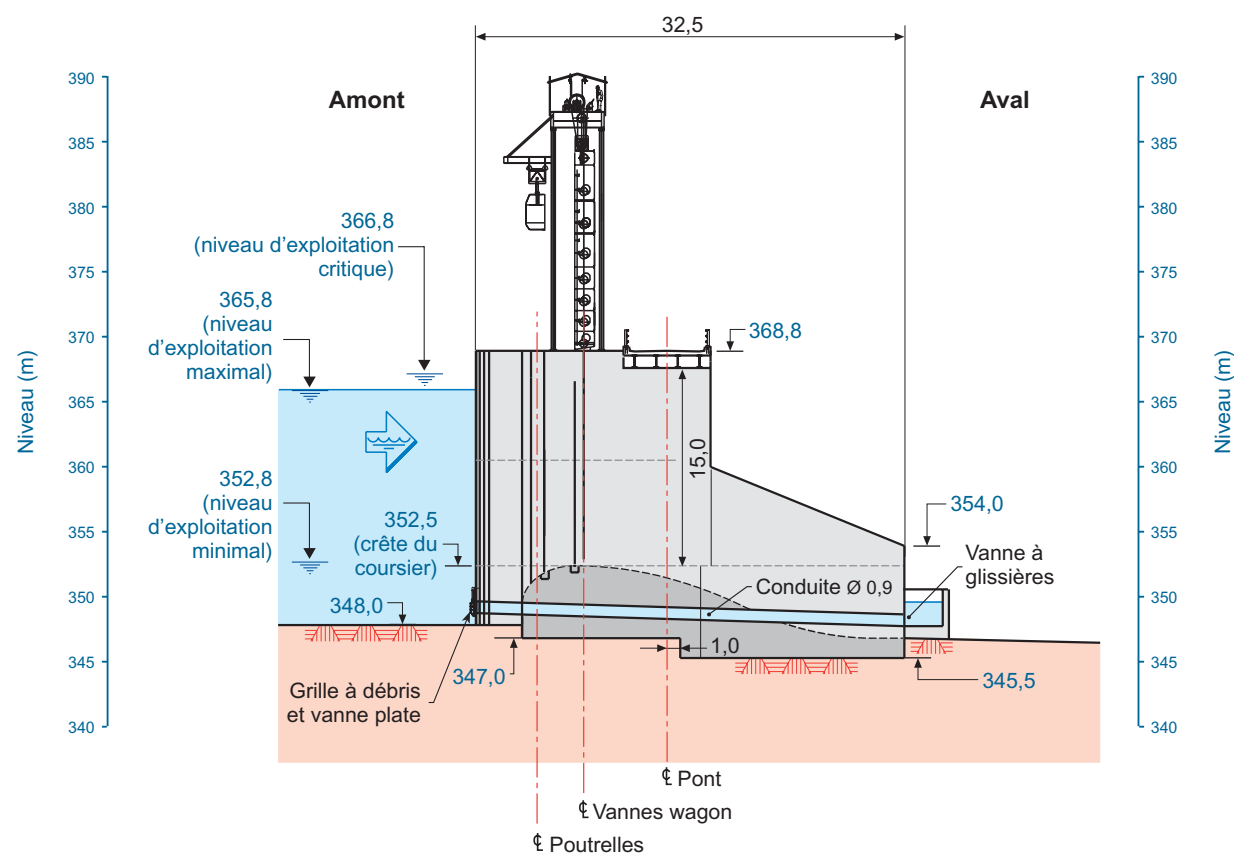
Évacuateur de crues – Détail
